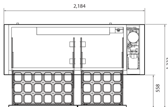
ВИД СВЕРХУ
